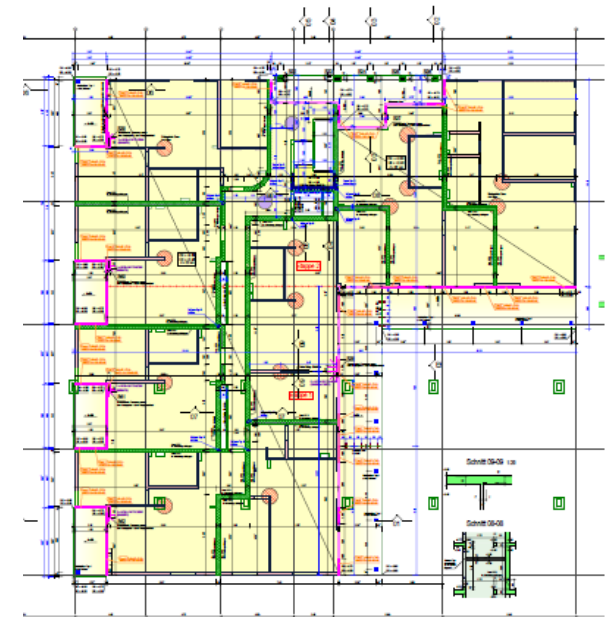
Schalung Wände und Decke EG
