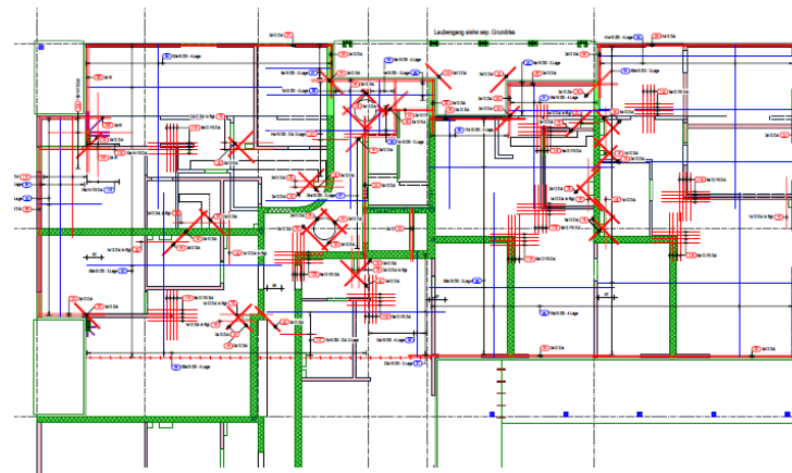
Bewehrung obere Lage, Decke 2. OG
