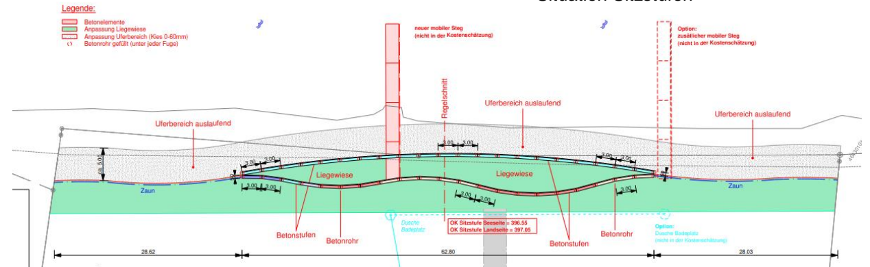
Situation Sitzstufen
