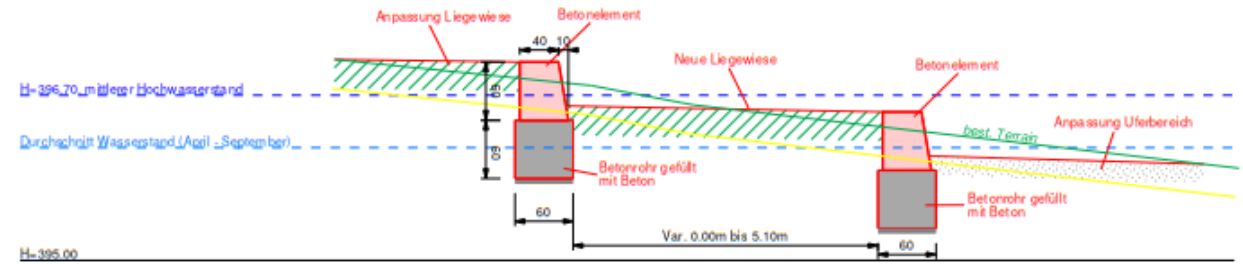
Situation Sitzstufen
