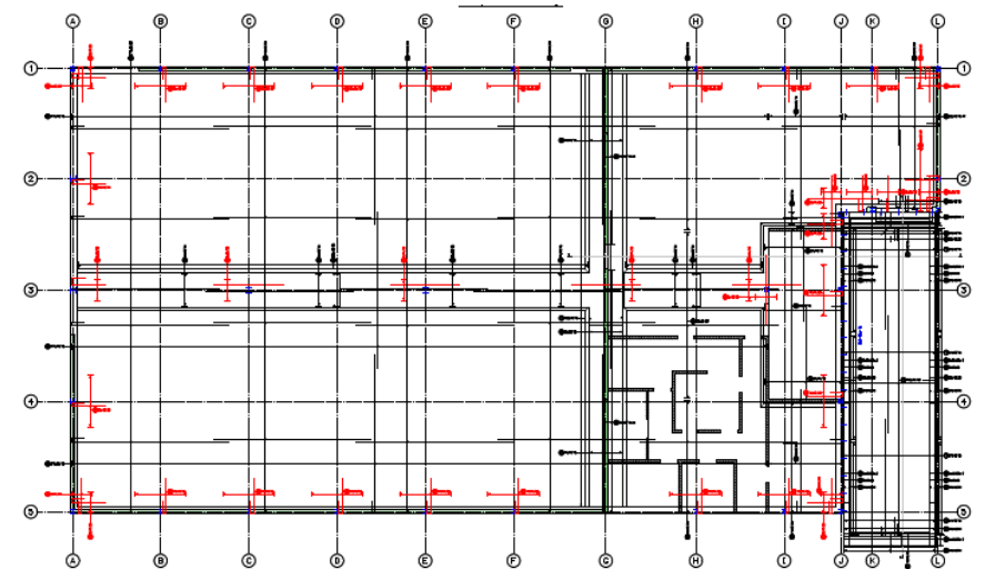
Bodenplatte Bewehrung untere Lage
