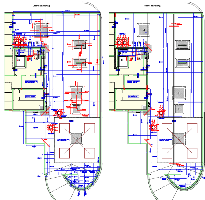
Bewehrung Bodenplatte
