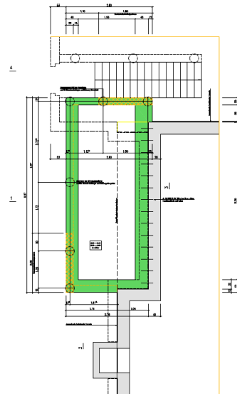
UG Schalung Grundriss Balkonturm
