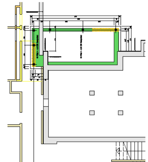
Mikropfähle Balkonturm
