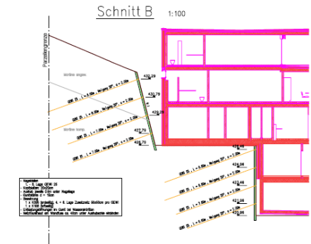
Baugrubensicherung Bodennägel
