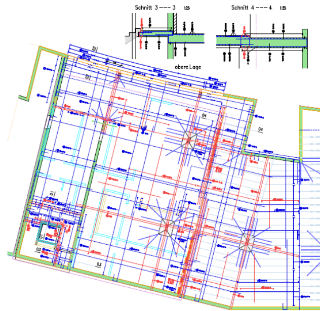
Armierung Decke UG
