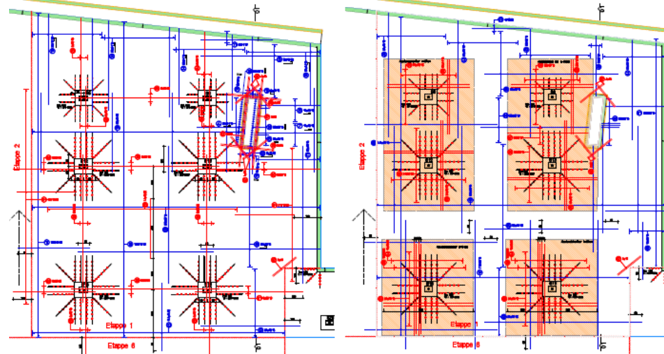
untere Lage - Grundriss Bewehrung Decke UG - obere Lage
