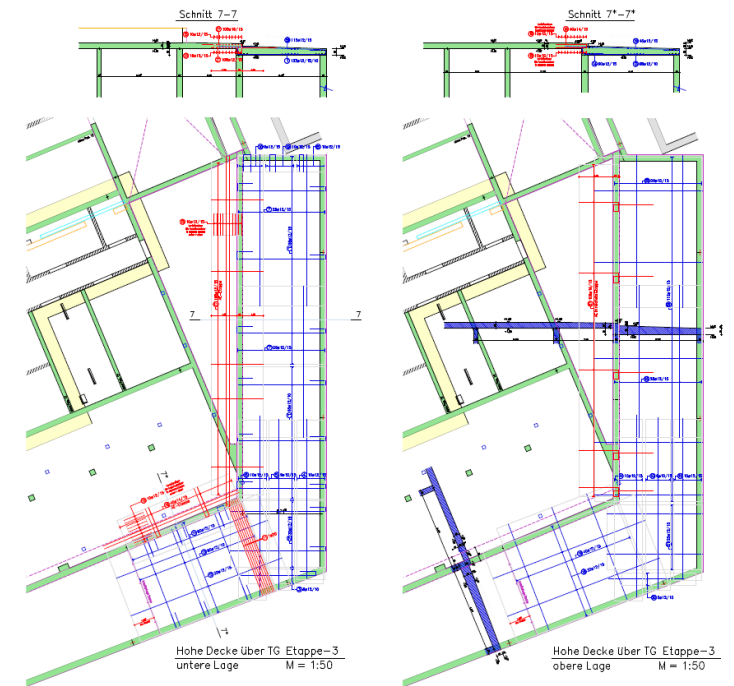
Bewehrung Hohe Decke über Tiefgarage
