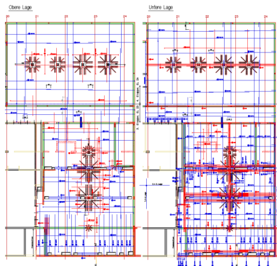
Decke Untergeschoss Bewehrung 3.+4. Etappe
