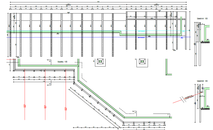
Rühlwände Nord Grundrisse und Ansichten
